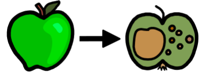
rots
