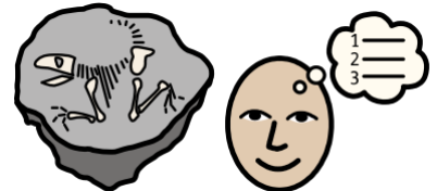
fossilisation
